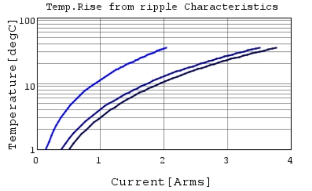
GCM21BR71E225KA73 Temp.rise — 100kHz —
