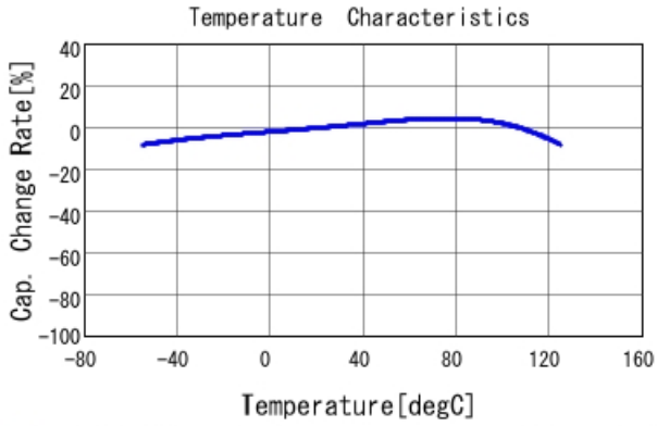
GCM21BR71A106KE22 C-Temp. capchange, DCO. 0V, ACO. 5Vrm
