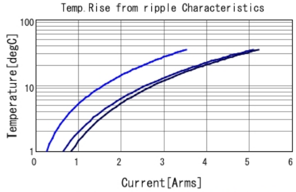
GCM21BR71A106KE22 Temp. rise ■ 80kHz ■ 400kHz ■ 800kHz
