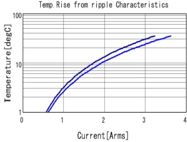
■ GCM21BC72A105KE36 Temp. rise ■ 500kHz ■ 1MHz
