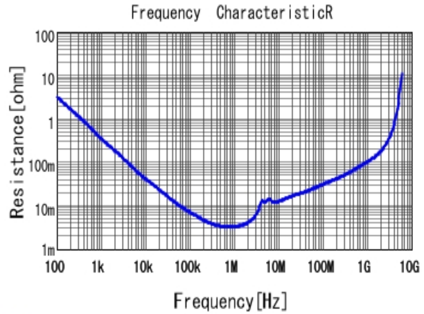
■ GCM21BC71C106KE36 R DCOV, 25degC
