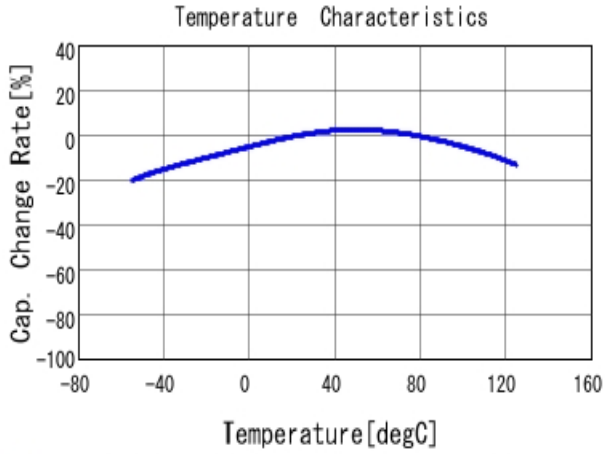
■ GCM21BC71C106KE36 C-Temp. capchange, DCO. 0V, ACO. 2V rm
