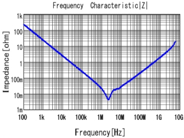
■ GCM21BC71C106KE36 |Z| DCOV, 25degC
