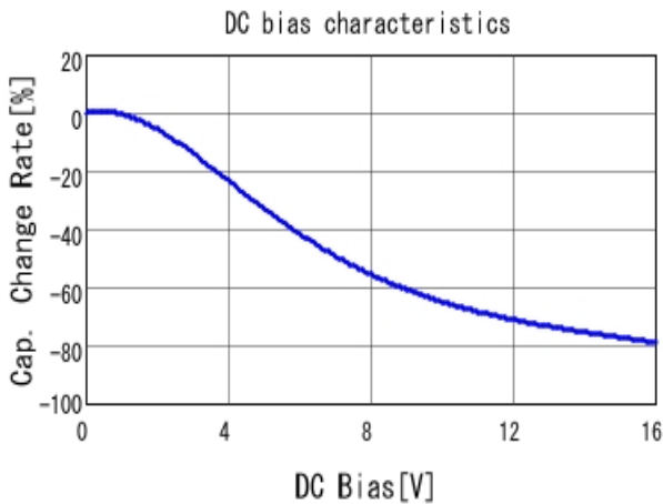
■ GCM21BC71C106KE36 C-DC bias capchange, 25.0degC, AC1V
