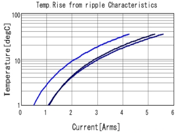
■ GCM21BC71C106KE36 Temp. rise ■ 80kHz ■ 400kHz ■ 800kHz
