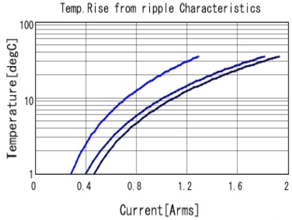
■ GCM188R71H104KA57 Temp. rise ■ 400kHz ■ 800kHz ■ 1MHz
