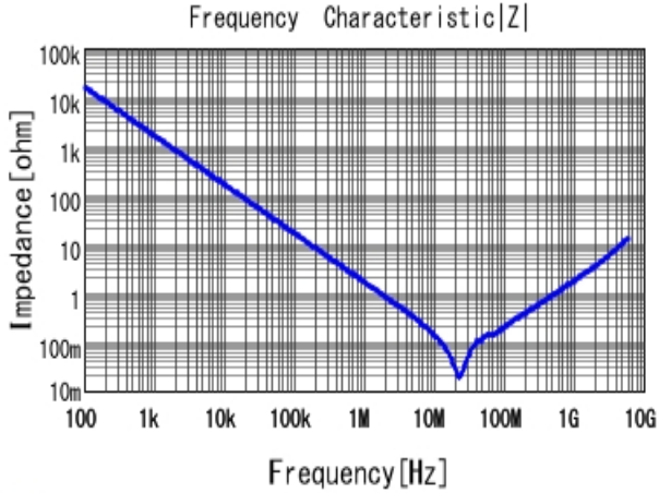
■ GCM188R71H104KA57 |Z| DC0V, 25degC
