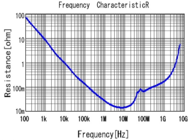
■ GCM188R71H104KA57 R DC0V, 25degC
