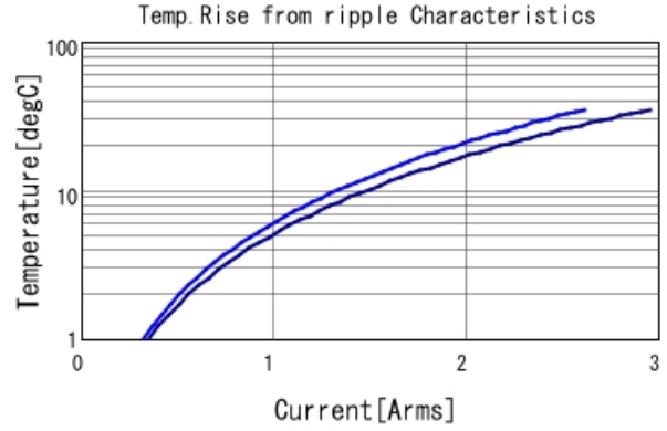
GCM188R71E105KA64 Temp. rise — 500kHz — 1MHz
