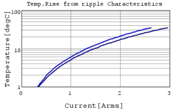
GCM188R71E105KA64 Temp.rise — 500kHz
