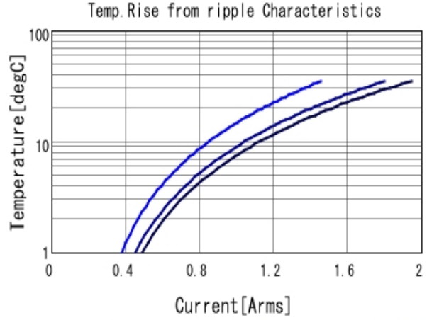
GCM188R71C334KA37 Temp. rise ■ 300kHz ■ 600kHz ■ 1MHz
