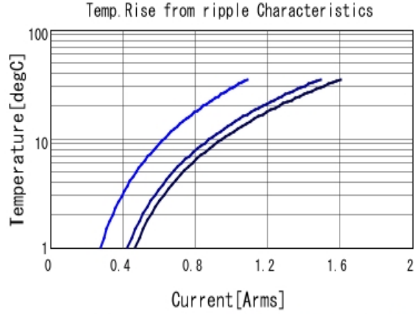
GCM188R71C104KA37 Temp. rise ■ 400kHz ■ 800kHz ■ 1MHz
