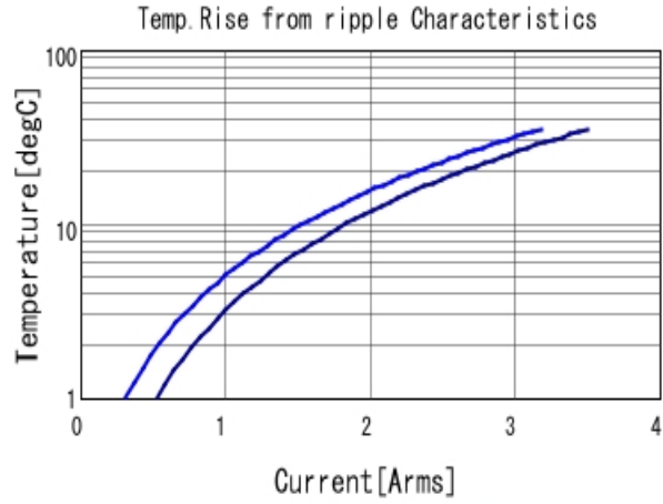
GCM188R70J225KE22 Temp. rise ■ 500kHz ■ 1MHz
