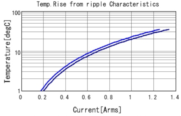
GCM155R71H104KE02 Temp. rise — 800kHz — 1MHz
