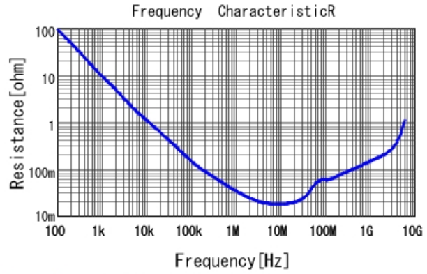
GCM155R71H104KE02 R DCOV, 25degC
