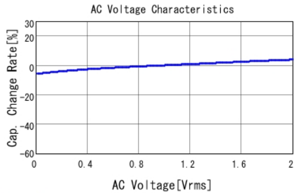
GCM155R71H104KE02 C-AC Voltage capchange, DCOV, 25
