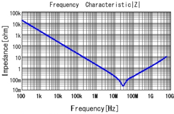
GCM155R71H104KE02 |Z| DCOV, 25degC
