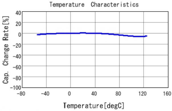
■ GCM155R71H103KA55 C-Temp. capchange, DCO. 0V, AC1. 0Vrm
