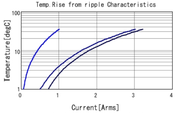
GCM155R71C224KE02 Temp. rise — 300kHz — 600
