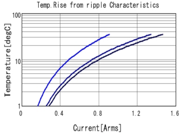
GCM155R71C104KA55 Temp. rise ■ 400kHz ■ 800kHz ■ 1MHz
