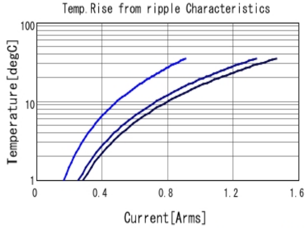
GCM155R71C104KA55 Temp. rise ■ 400kHz ■ 800kHz ■ 1MHz
