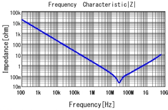
GCM155L8EH104KE07 |Z| DC0V, 25degC
