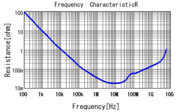
GCM155L8EH104KE07 R DC0V, 25degC
