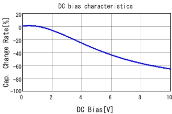
GCM155C71A684KE38 C-DC bias capchange, 25.0degC, AC1V
