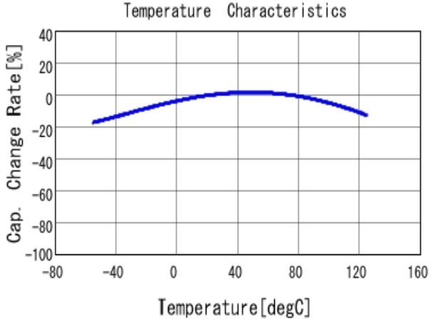
GCM155C71A474KE36 C-Temp. capchange, DCO. 0V, ACO. 2V rm
