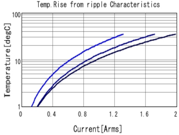
GCM155C71A474KE36 Temp. rise ■ 200kHz ■ 500kHz ■ 1MHz
