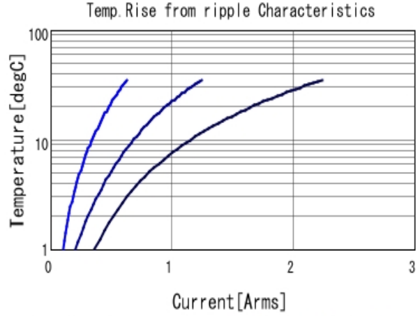
GCJ43DR72J104KXJ1 Temp. rise 30kHz 100kHz 300kHz
