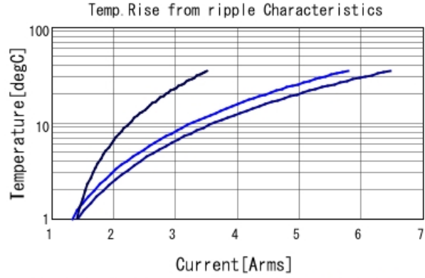
GCJ32EC71H106KA01 Temp. rise ■ 80kHz ■ 400kHz ■ 800kHz
