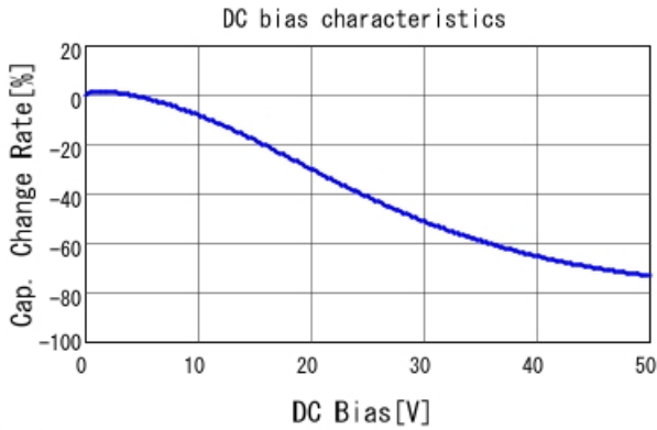
■ GCJ32EC71H106KA01 C-DC bias capchange, 25.0degC, AC1.
