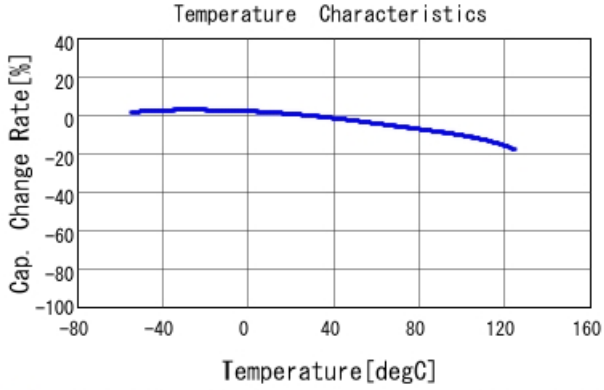
■ GCJ32EC71H106KA01 C-Temp. capchange, DCO. 0V, AC1. 0Vrm
