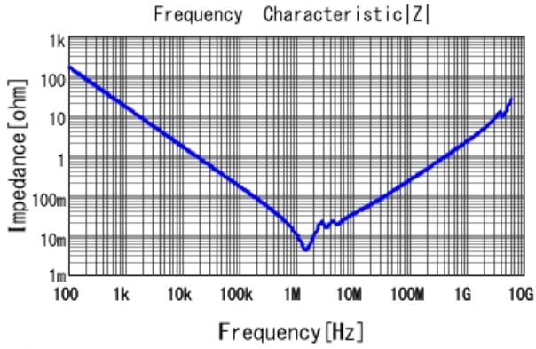
■ GCJ32EC71H106KA01 |Z| DC0V, 25degC
