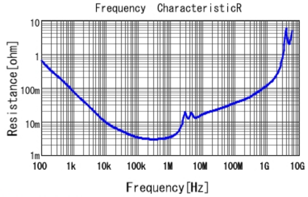
■ GCJ32EC71H106KA01 R DC0V, 25degC
