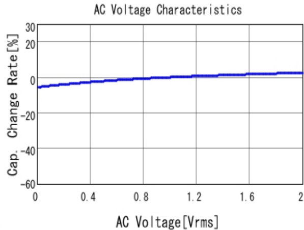
■ GCJ31CC71E106KA15 C-AC Voltage capchange, DC0V, 25.0d
