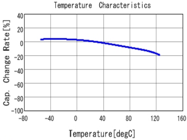
■ GCJ31CC71E106KA15 C-Temp. capchange, DCO. 0V, AC1.0V rm
