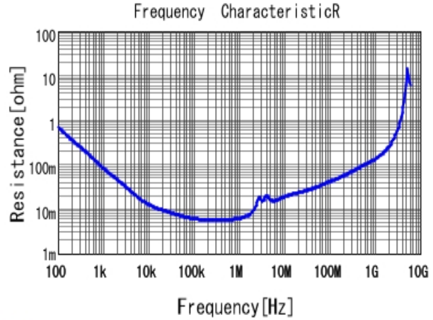
■ GCJ31CC71E106KA15 R DC0V, 25degC
