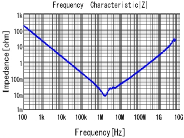
■ GCJ31CC71E106KA15 |Z| DC0V, 25degC
