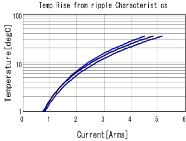
GCJ31CC71E106KA15 Temp. rise ■ 80kHz ■ 400kHz ■ 800kHz
