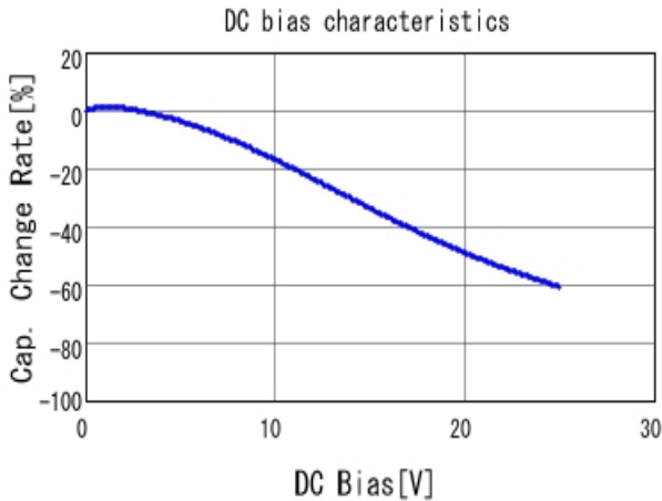
■ GCJ31CC71E106KA15 C-DC bias capchange, 25.0degC, AC1.
