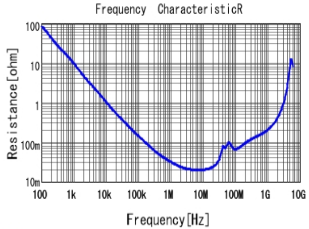
■ GCJ21BR72A104KA01 R DCOV, 25degC
