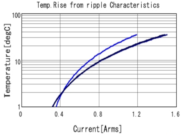
GCJ21BR72A104KA01 Temp. rise ■ 400kHz ■ 800kHz ■ 1MHz
