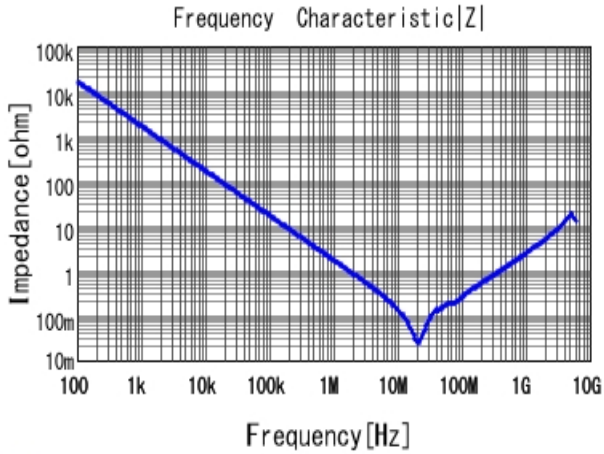
■ GCJ21BR72A104KA01 |Z| DCOV, 25degC
