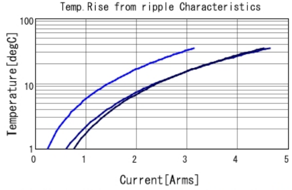
GCJ21BR71C475KA01 Temp. rise ■ 100kHz ■ 500kHz ■ 1MHz
