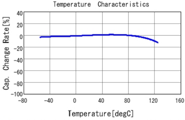
■ GCJ21BR71C475KA01 C-Temp. capchange, DCO. 0V, AC1. 0Vrm
