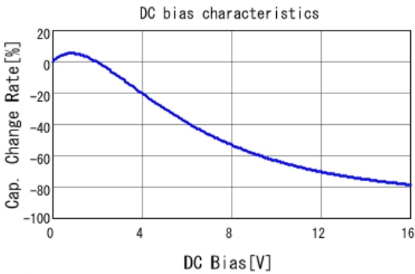
■ GCJ21BR71C475KA01 C-DC bias capchange, 25.0degC, AC1.
