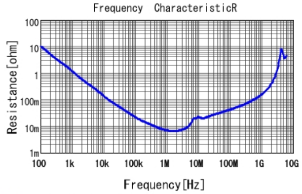
■ GCJ21BR71C475KA01 R DC0V, 25degC
