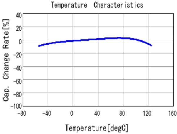
■ GCJ21BR71A106KE01 C-Temp. capchange, DCO. 0V, ACO. 5V rm
