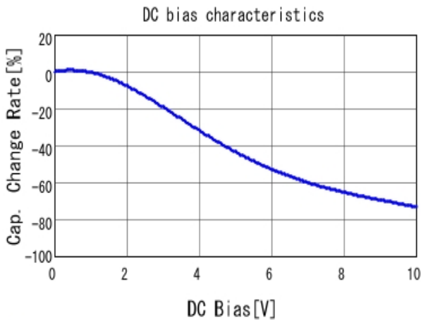
■ GCJ21BR71A106KE01 C-DC bias capchange, 25.0degC, AC1V
