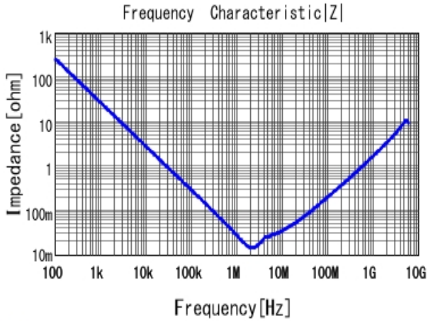
■ GCJ21BR71A106KE01 |Z| DCOV, 25degC
