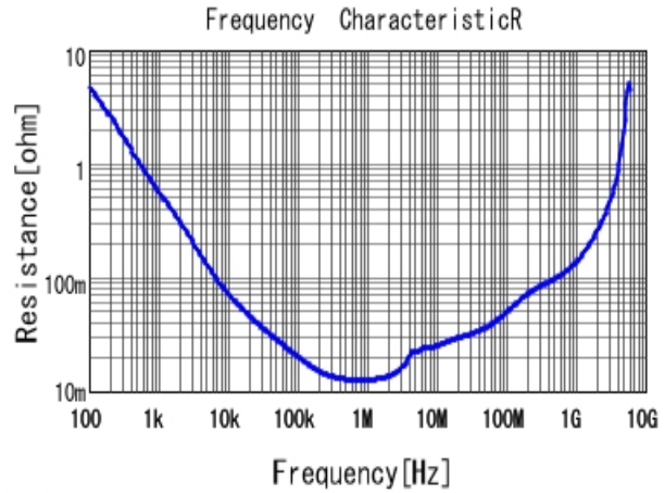
■ GCJ21BR71A106KE01 R DCOV, 25degC
