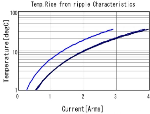
GCJ21BR71A106KE01 Temp. rise ■ 80kHz ■ 400kHz ■ 800kHz
