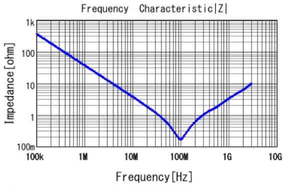
■ GCJ21AR72E472KXJ1 |Z| DC0V, 25degC
