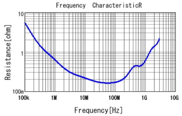
■ GCJ21AR72E472KXJ1 R DC0V, 25degC
