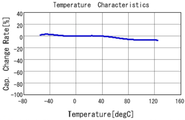
■ GCJ188R72A103KA01 C-Temp. capchange, DCO. 0V, AC1. 0Vrm
