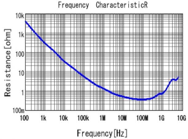
■ GCJ188R71H222KA01 R DCOV, 25degC
