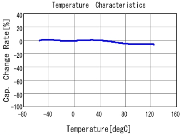
■ GCJ188R71H222KA01 C-Temp. capchange, DCO. 0V, AC1. 0Vrm
