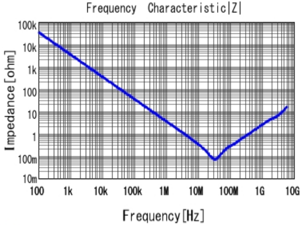
■ GCJ188R71E473KA01 |Z| DCOV, 25degC
