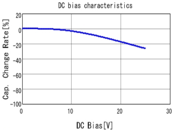
■ GCJ188R71E473KA01 C-DC bias capchange, 25.0degC, AC1.
