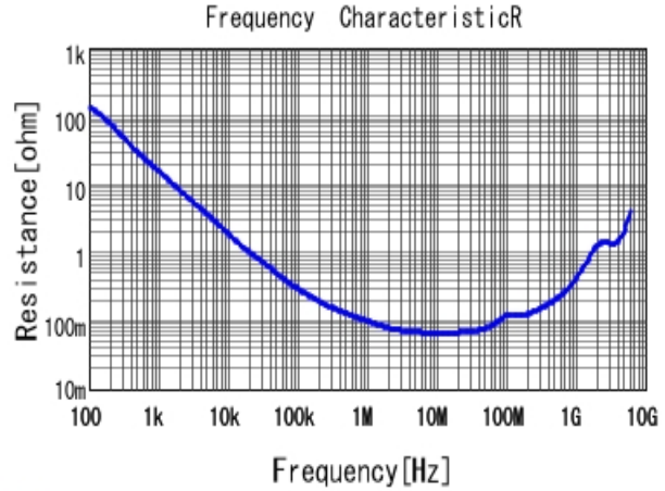
■ GCJ188R71E473KA01 R DCOV, 25degC
