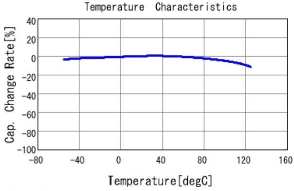
■ GCJ188R71E105KA01 C-Temp. capchange, DCO. 0V, AC1. 0Vrm
