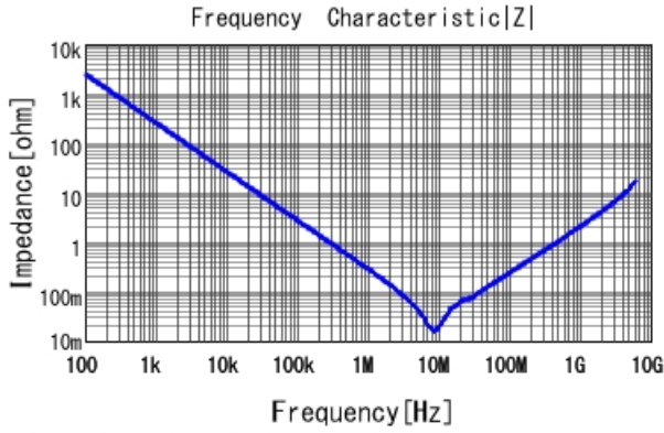
■ GCJ188R71E105KA01 |Z| DC0V, 25degC
