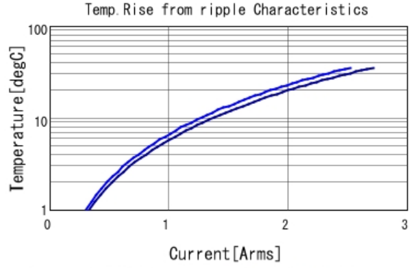
GCJ188R71E105KA01 Temp. rise ■ 500kHz ■ 1MHz
