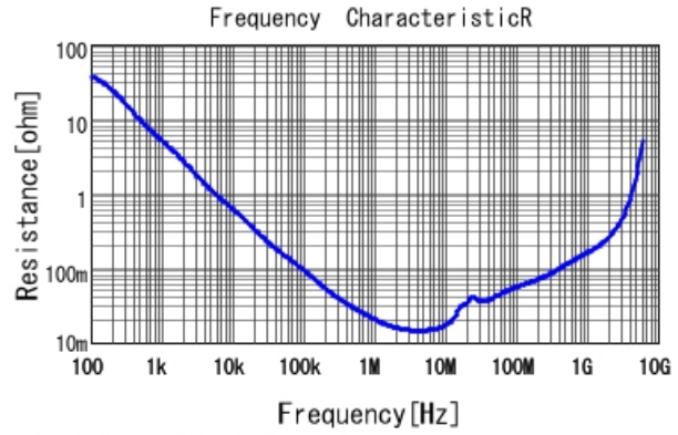
■ GCJ188R71E105KA01 R DC0V, 25degC
