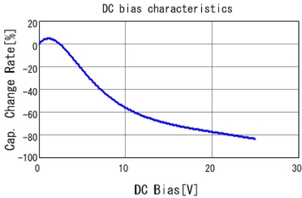
■ GCJ188R71E105KA01 C-DC bias capchange, 25.0degC, AC1.
