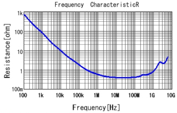
■ GCJ188R71E103KA01 R DCOV, 25degC
