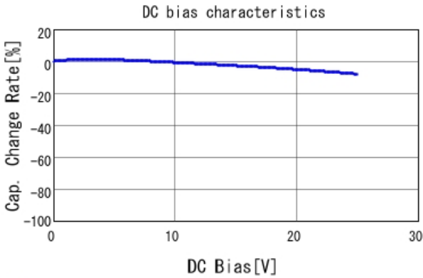
■ GCJ188R71E103KA01 C-DC bias capchange, 25.0degC, AC1.
