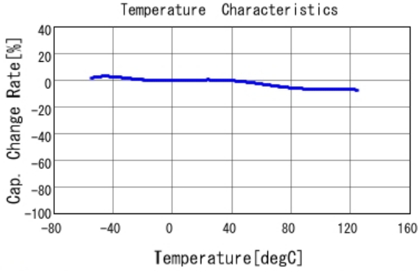
■ GCJ188R71E103KA01 C-Temp. capchange, DCO. 0V, AC1. 0Vrm
