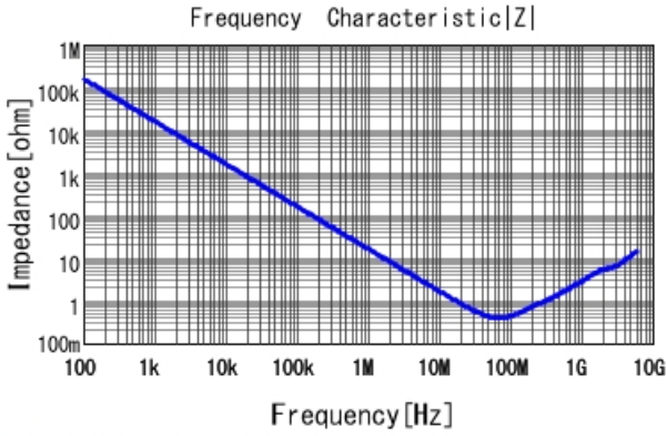
■ GCJ188R71E103KA01 |Z| DCOV, 25degC
