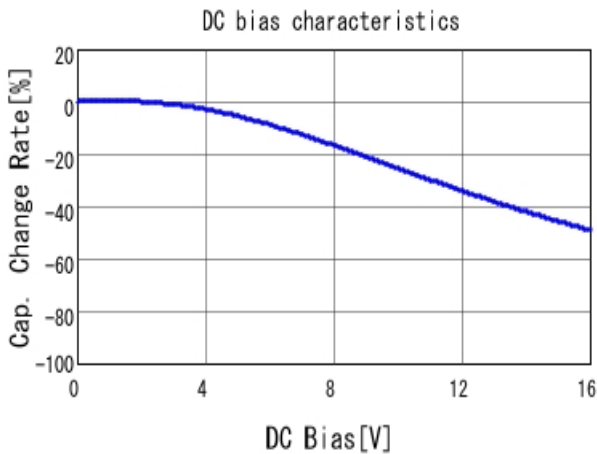
■ GCJ188R71C474KA12 C-DC bias capchange, 25.0degC, AC1.
