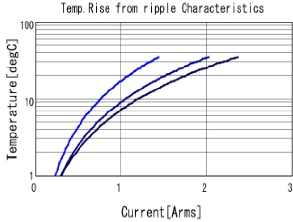
GCJ188R71C474KA12 Temp. rise ■ 200kHz ■ 500kHz ■ 1MHz
