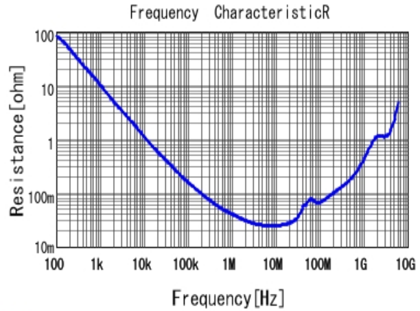
■ GCJ188R71C104KA01 R DCOV, 25degC
