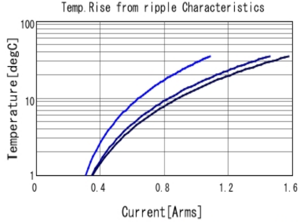
GCJ188R71C104KA01 Temp. rise ■ 400kHz ■ 800kHz ■ 1MHz
