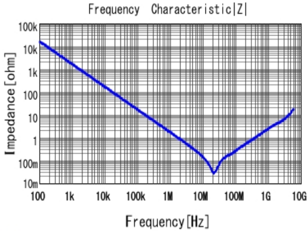
■ GCJ188R71C104KA01 |Z| DCOV, 25degC
