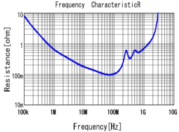
■ GA355QR7GF332KW01 R DCOV, 25degC
