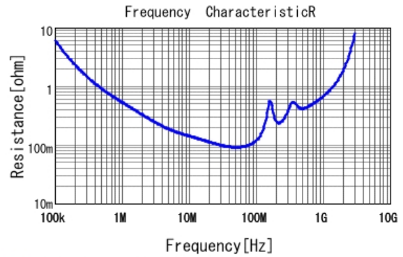
■ GA343DR7GD472KW01 R DCOV, 25degC
