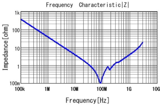
■ GA343DR7GD472KW01 |Z| DCOV, 25degC
