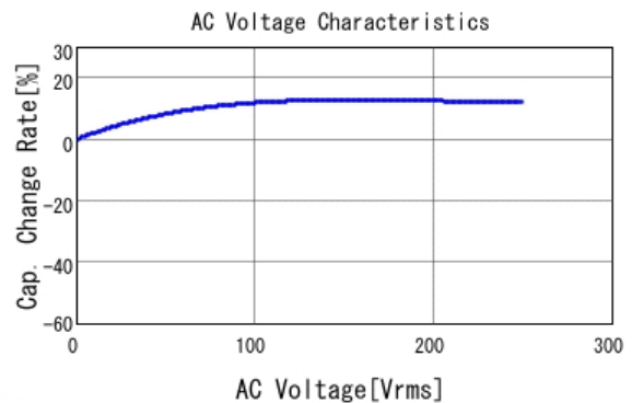
■ GA343DR7GD472KW01 C-AC Voltage capchange, DCOV, 25.0d
