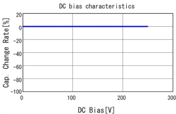
■ GA343DR7GD472KW01 C-DC bias capchange, 25.0degC, AC1V
