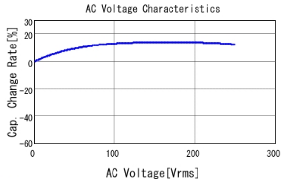
■ GA342QR7GD152KW01 C-AC Voltage capchange, DCOV, 25.0d
