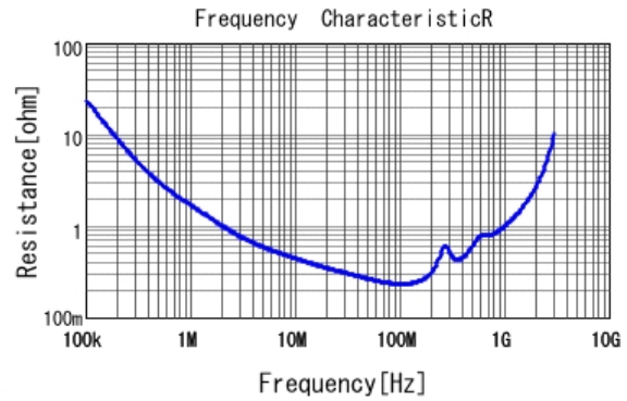
■ GA342QR7GD152KW01 R DCOV, 25degC
