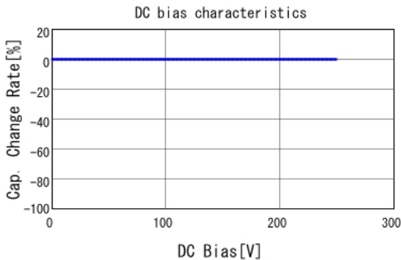
■ GA342QR7GD152KW01 C-DC bias capchange, 25.0degC, AC1V
