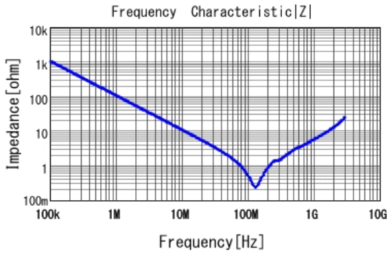
■ GA342QR7GD152KW01 |Z| DCOV, 25degC
