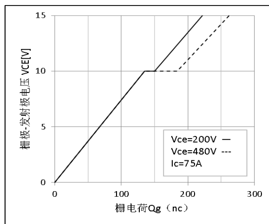
图 18 栅电荷特性
