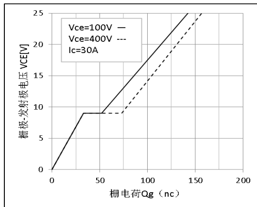
图 18 栅电荷特性
