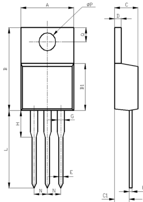
外形图: CRG20T60A83L (TO-220)
