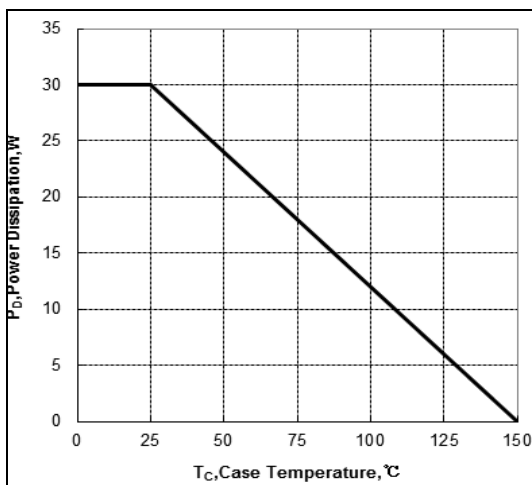
图 17 耗散功率-壳温 Tc 特性 (220AB)
