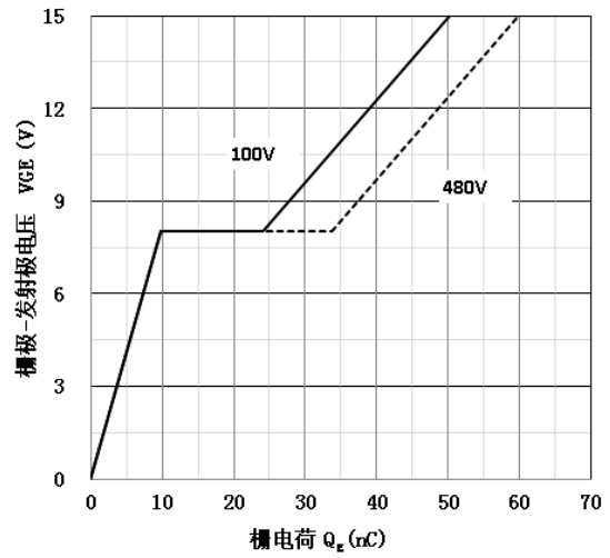
图 14.栅电荷特性
