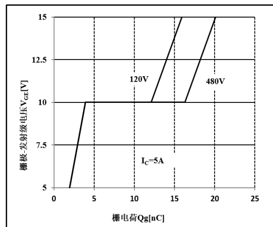
图 18 栅电荷特性
