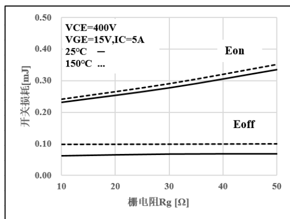
图 6 开关损耗-栅电阻特性曲线
