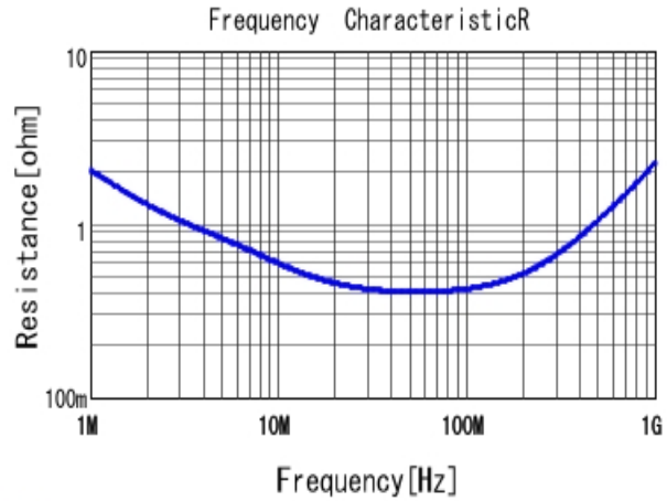
■ DE2E3SA222MA3BY02F R DCOV, 20degC
