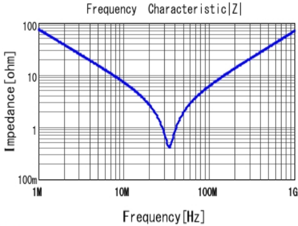
■ DE2E3SA222MA3BY02F |Z| DCOV, 20degC
