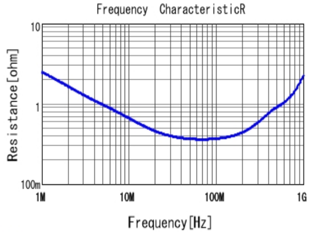
■ DE2E3SA222MA3BT02F R DCOV, 20degC
