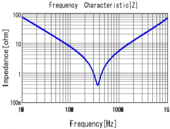
■ DE2E3SA222MA3BT02F |Z| DCOV, 20degC
