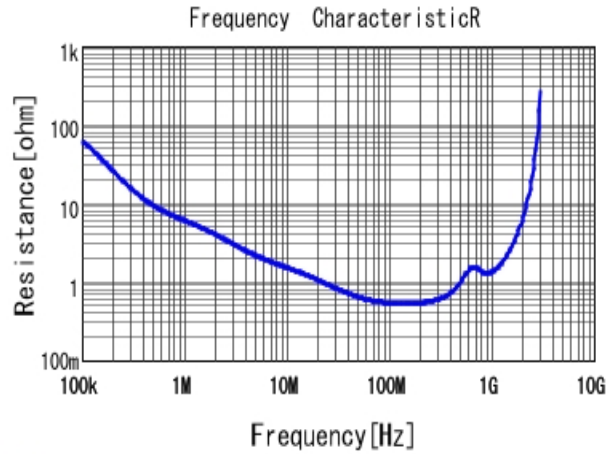
■ DE2E3KY102MB2BM01F R DCOV, 20degC
