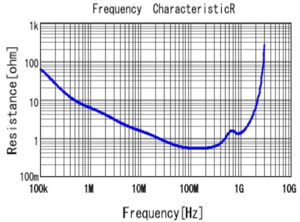
■ DE2E3KY102MA2BM01F R DCOV, 20degC
