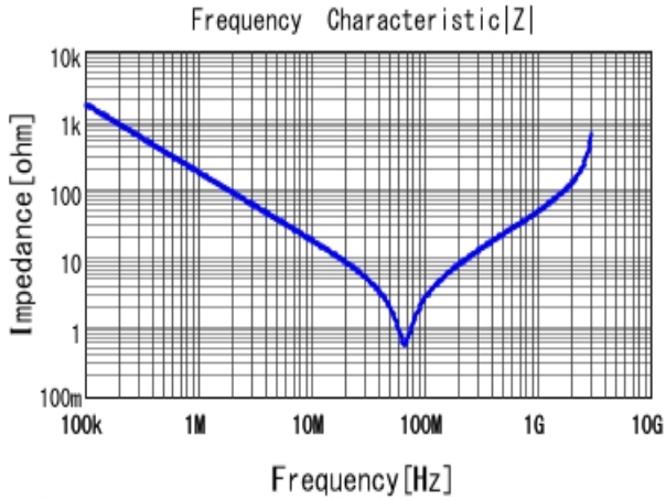
■ DE2E3KY102MA2BM01F |Z| DCOV, 20degC
