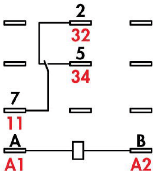
SPDT
