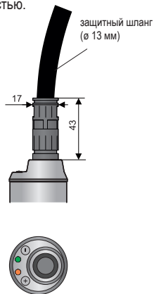
Исполнение «Н» с выводом для защитного шланга - для применения в наружной среде в местах с повышенной влажностью.
