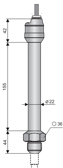
Исполнение «С» с разъемом M12
