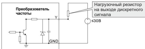
а) Схема подключения нагрузочного резистора к выходу дискретного сигнала
