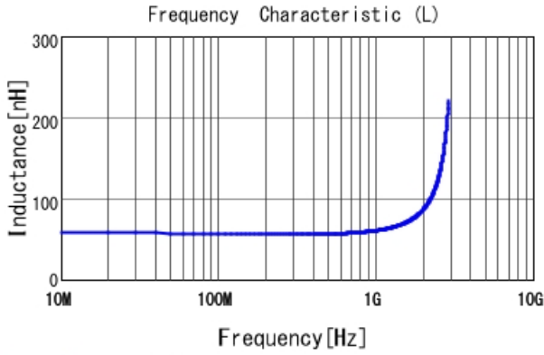
LQW15AN56NG00 L
