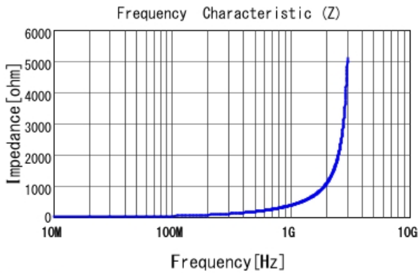
LQW15AN56NG00 |Z|
