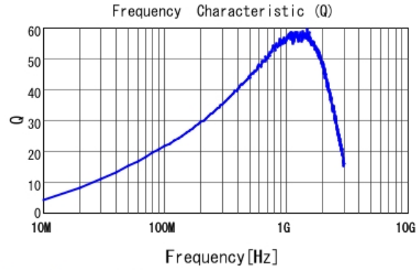
LQW15AN56NG00 Q
