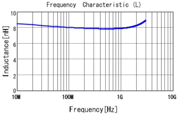
■ LQW15AN8N2G00 L
