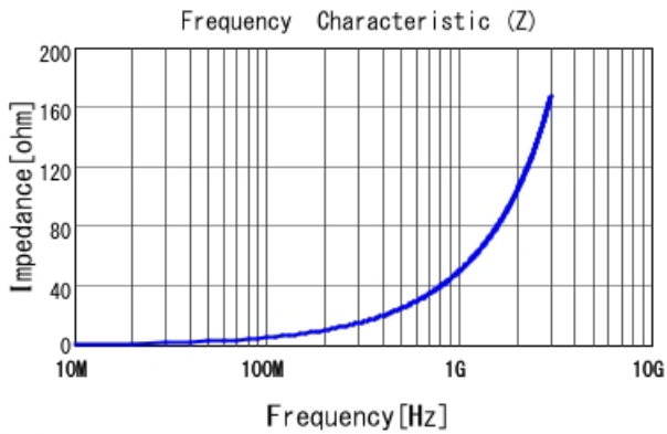
■ LQW15AN8N2G00 |Z|
