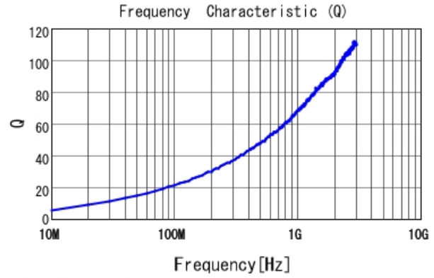
■ LQW15AN8N2G00 Q
