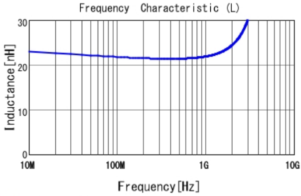
■ LQW15AN22NJ00 L
