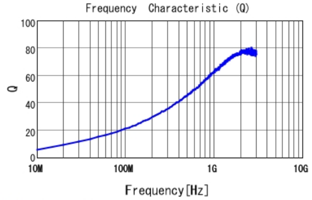
■ LQW15AN22NJ00 Q
