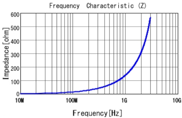
■ LQW15AN22NJ00 |Z|
